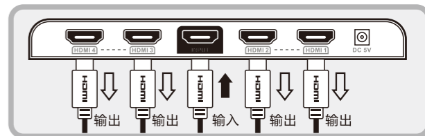
将一路HDMI信号分配成四路HDMI信号
